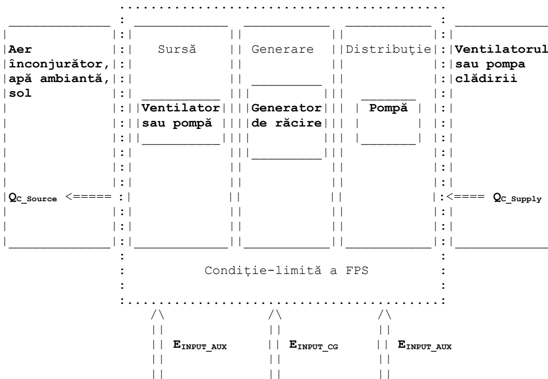
Figura 1 Ilustrarea condițiilor-limită ale FPS pentru generatorul de răcire care utilizează FPS standard și răcirea centralizată (și alte sisteme de răcire de dimensiuni mari care utilizează FPS măsurat), unde E_{INPUT\_AUX} este energia de intrare pentru ventilator și/sau pompă și E_{INPUT\_CG} energia de intrare pentru generatorul de răcire
